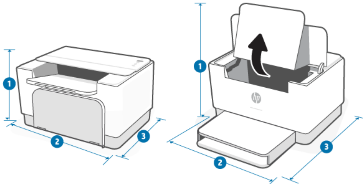
Abbildung A-1 Abmessungen des Druckers
